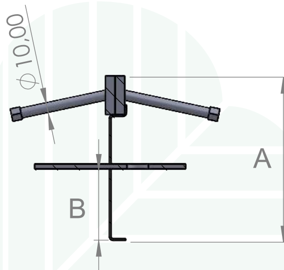
РАЗРЕЗ С - С МАЩАБ 1 : 5
